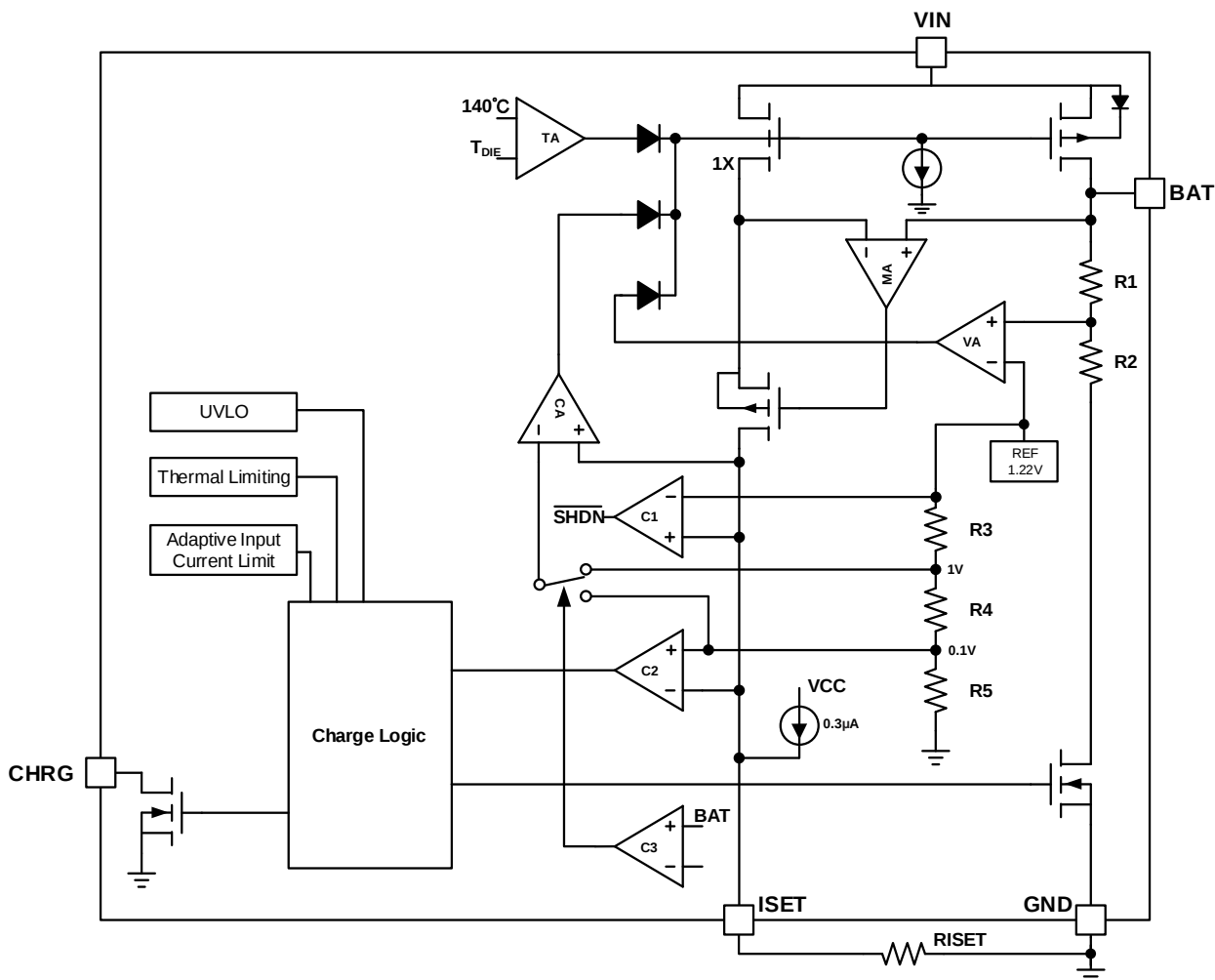
图 1. GD30BC1502 功能框图
