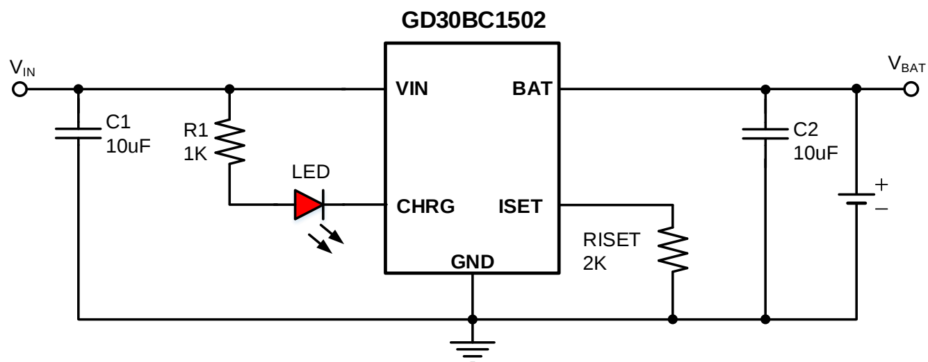
图 3. 480mA 恒流充电参考电路
